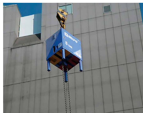
「無線操作反転吊り装置 写楽」 “写”は長い資材を斜めに吊るすことができるため“斜”からとった
